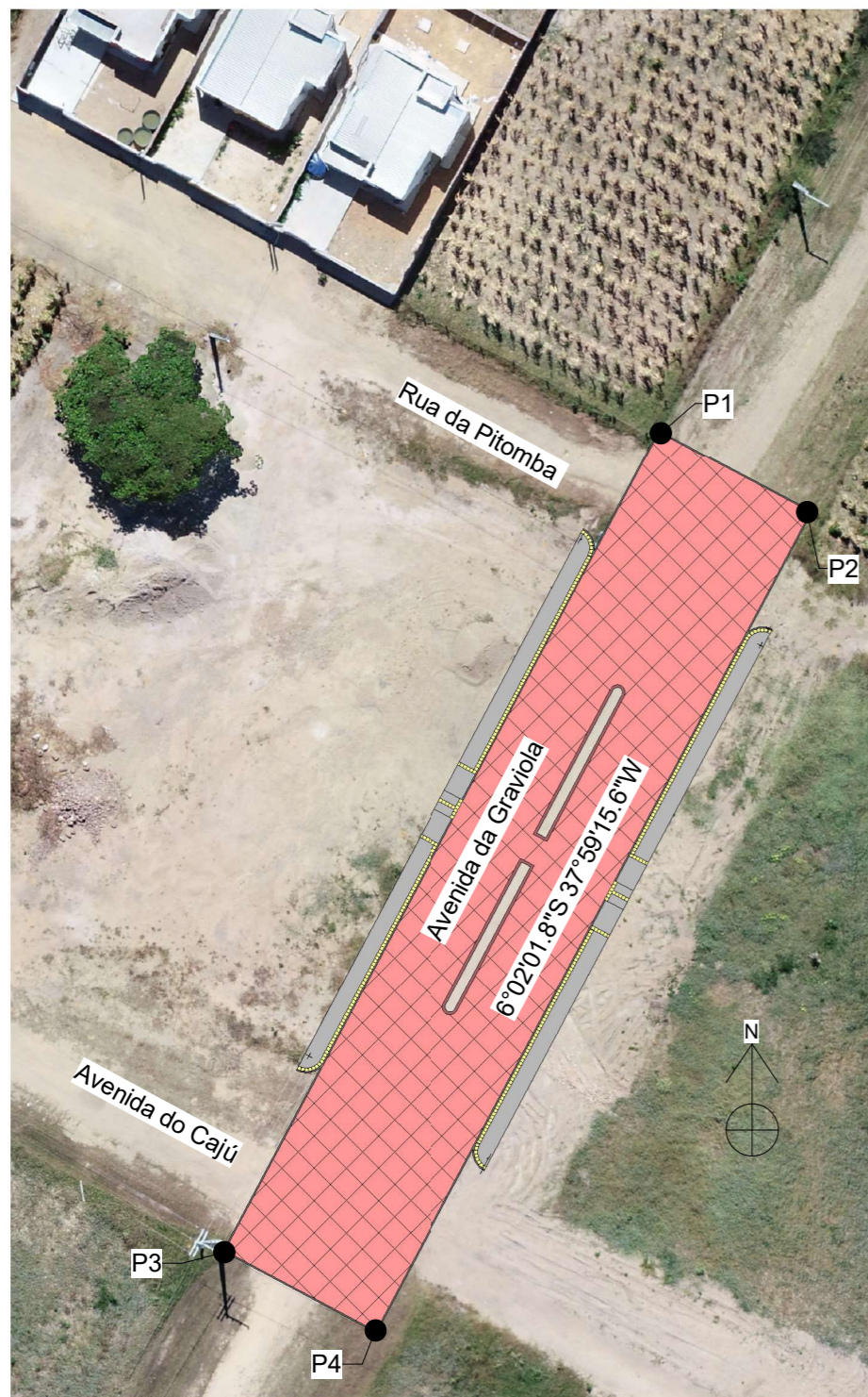
1 Planta de Localização AV Graviola 1 : 500
